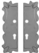
3417501 16x29,5cm, 2mm.
