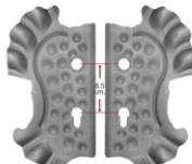
3417101 16x29cm, 2mm.
