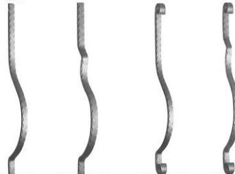
CODE Mz.Mak. Kg C-20501 20x10 1,41 C-20505 20x05 0,70 C-20501 20x10 1,77 C-20505 20x05 0,88 C-30501 30x10 2,12 C-30505 30x05 1,06
