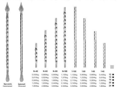
Nervürlü Hammered İşlemeli Grooved N-40 0,430kg N-60 0,680kg N-80 0,900kg N-100 1,130kg I-100 1,130kg I-80 0,900kg I-60 0,680kg I-40 0,430kg N-40 0,610kg N-60 0,924kg N-80 1,232kg N-100 1,579kg I-100 1,579kg I-80 1,232kg I-60 0,924kg I-40 0,610kg N-40 0,840kg N-60 1,260kg N-80 1,680kg N-100 2,110kg I-100 2,110kg I-80 1,680kg I-60 1,260kg I-40 0,840kg N-40 1,230kg N-60 1,830kg N-80 2,440kg N-100 3,140kg I-100 3,140kg I-80 2,440kg I-60 1,830kg I-40 1,230kg N-40 1,800kg N-60 2,680kg N-80 3,600kg N-100 4,520kg I-100 4,520kg I-80 3,600kg I-60 2,680kg I-40 1,800kg
