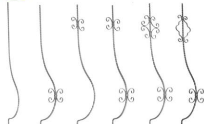
C-760 1,2x25,5x25 1,51kg
